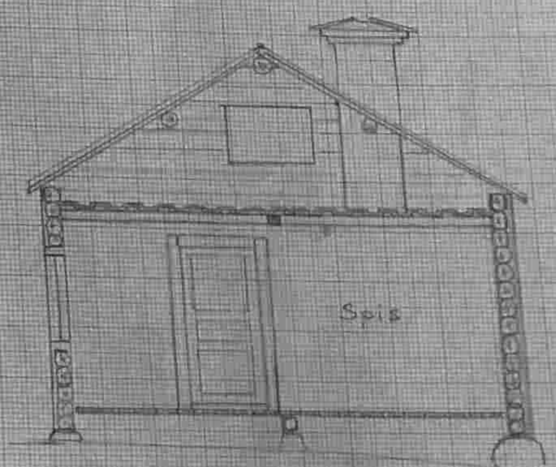
Skärning B-B
