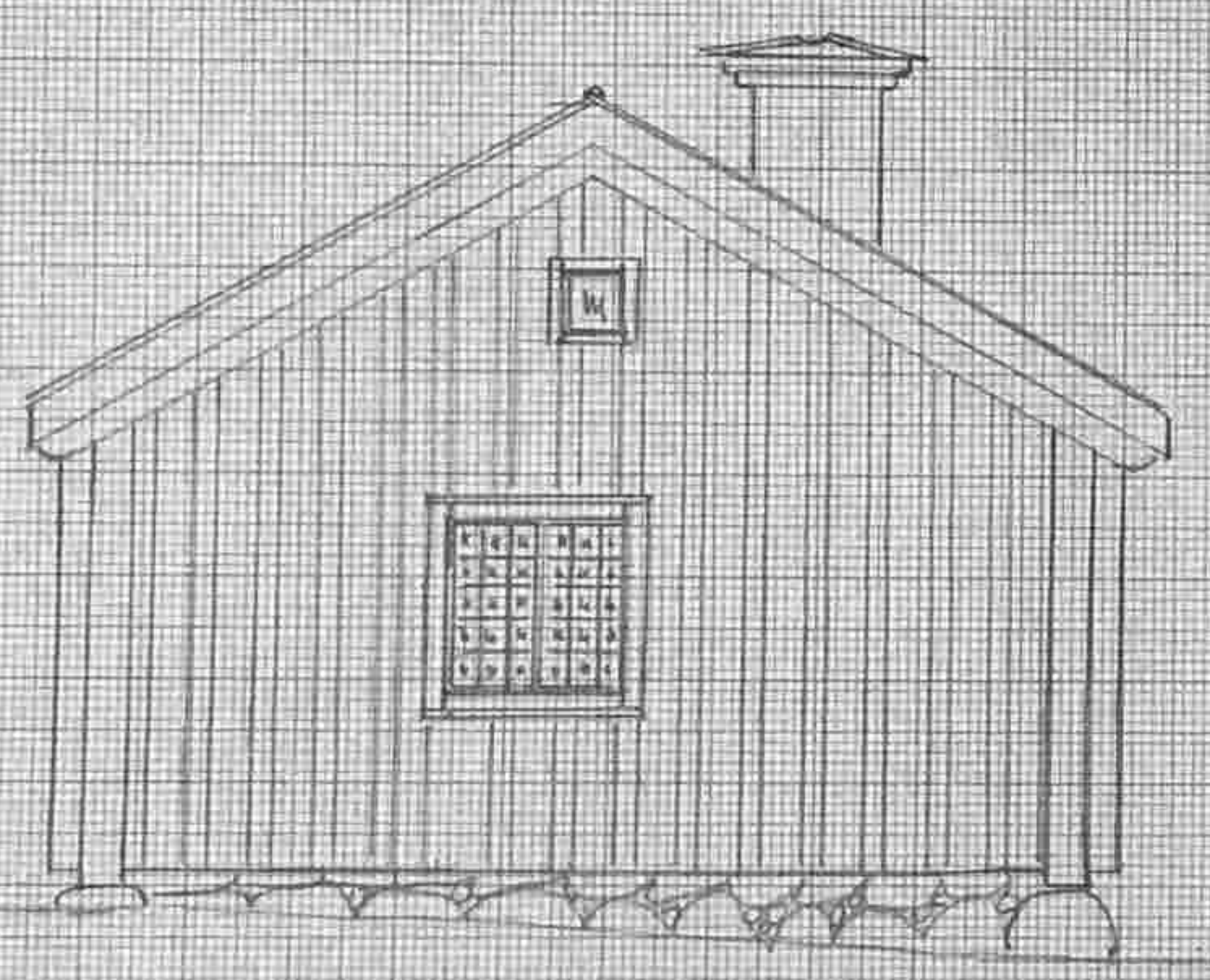
Fasad mot söder
